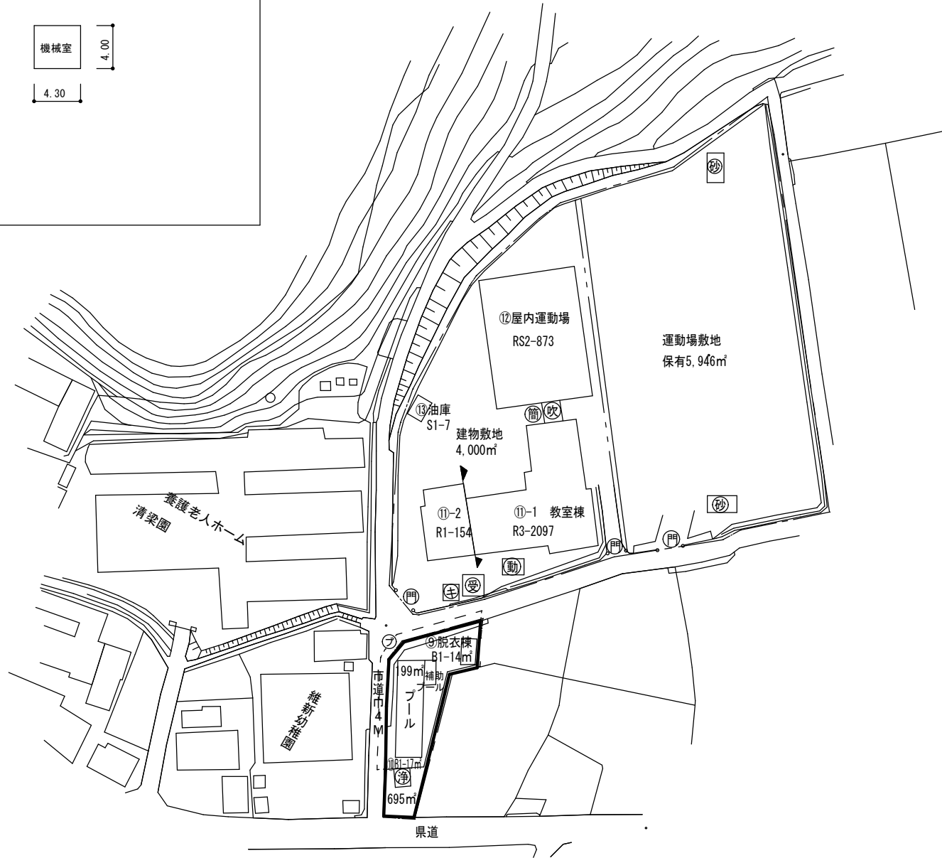
旧維新小学校プール配置図
