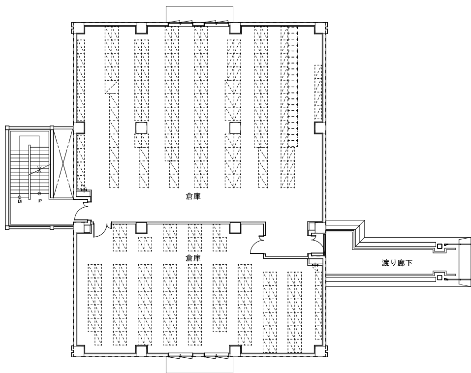
3階平面図
