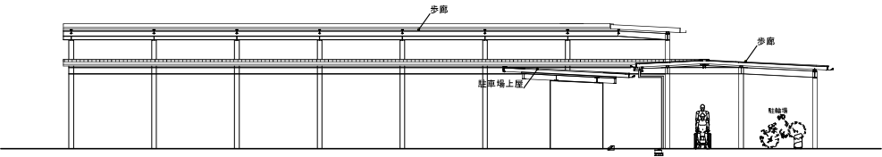
西立面図
