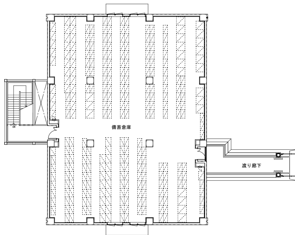
4階平面図
