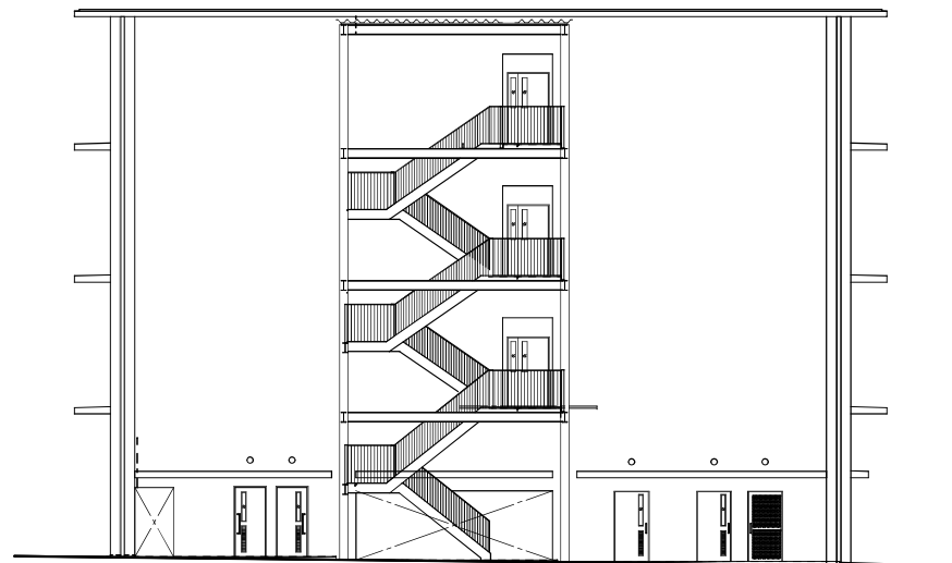
西立面图
