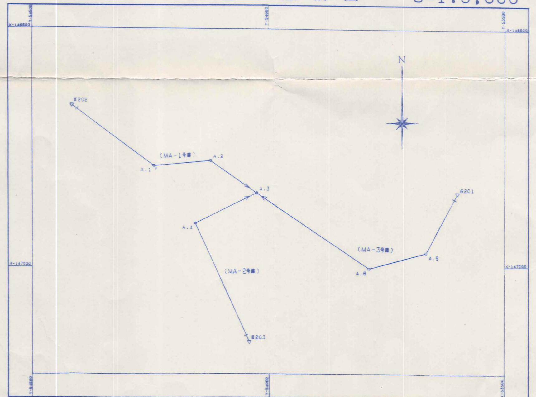
3級基準点網図
