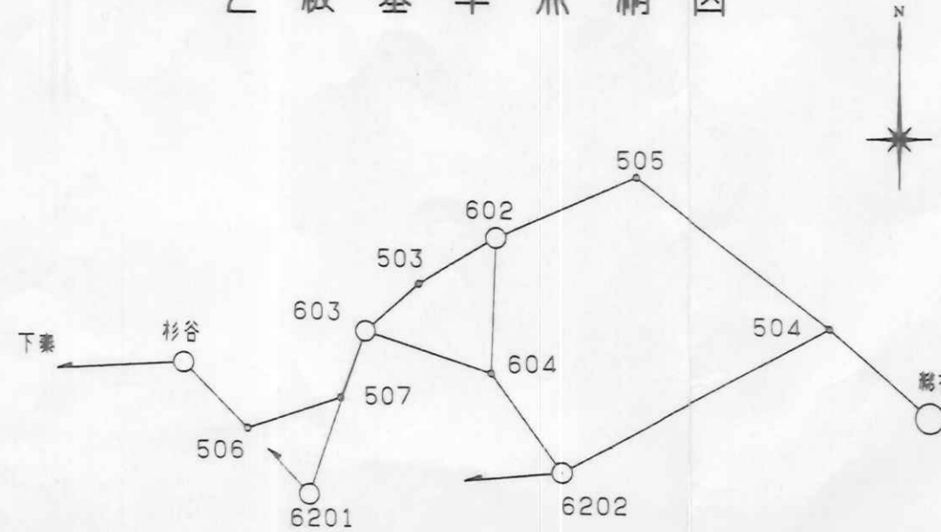
2級基準點網圖
