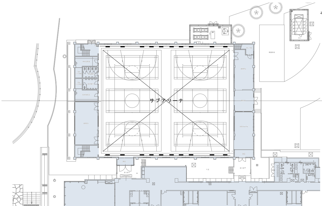
(サブアリーナ) 2階平面図
