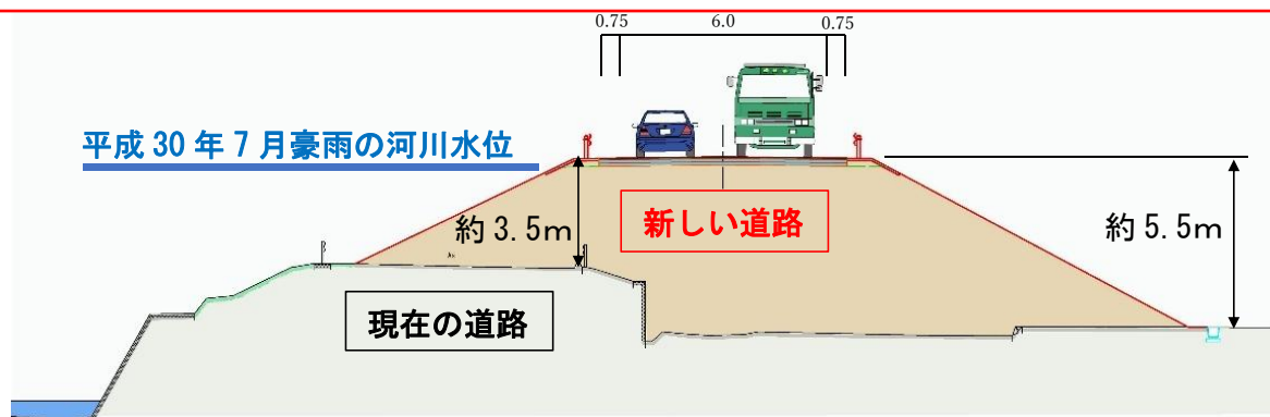
対策工事（堤防整備）イメージ
