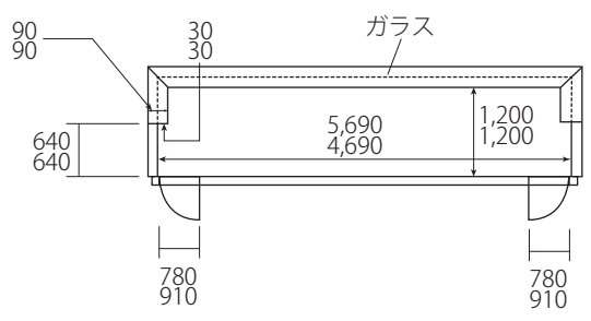
[展示ケース] (上段=中央、下段=両脇)
